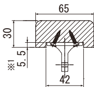
手摺形状例
