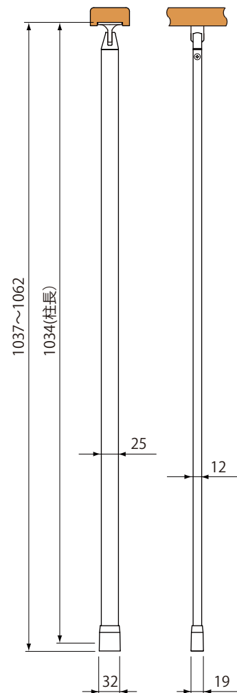
子支柱(991)セット
