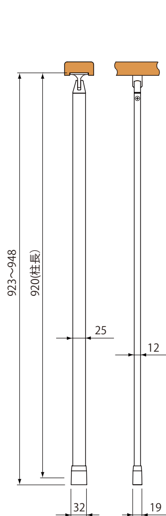
子支柱(877)セット
