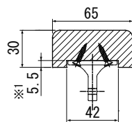
手摺形状例
