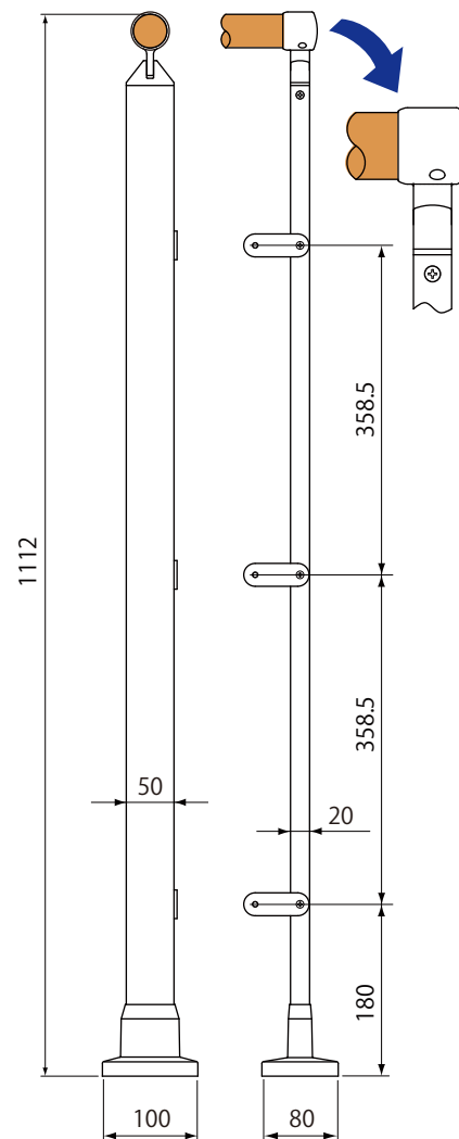
親支柱スタート用セット
