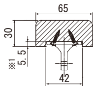
手摺形状例
