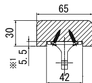
手摺形状例
